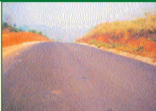
3 - Vista da Pavimentação da RO-010
